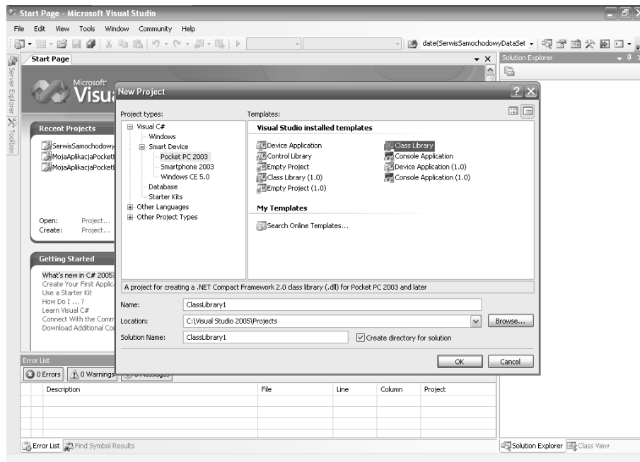
Rysunek 2 – Okno dialogowe wyboru nowego projektu (biblioteki łączącej dynamicznie – dll)
